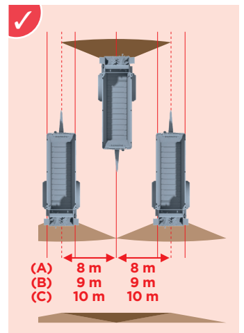
Largeurs de croisement (variables selon la matière épandue) : (A) 8 m (standard) (B) 9 m avec couteaux cuillères (C) 10 m avec plateaux d'épandage
